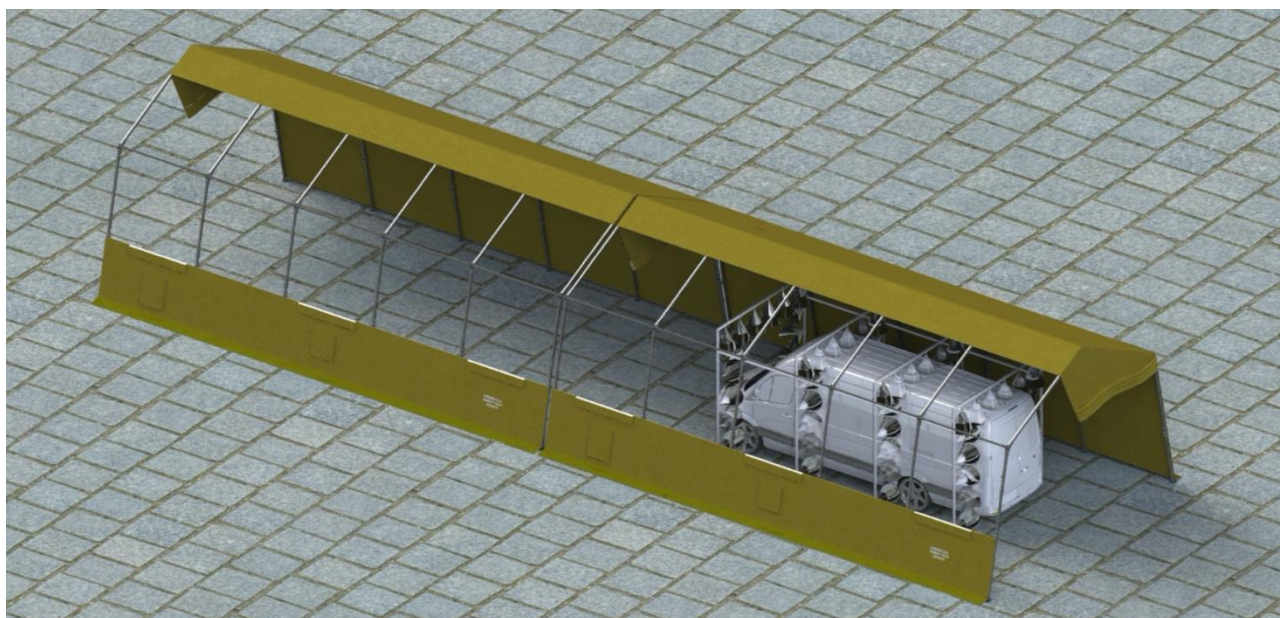
Wariant 1: dekontaminacja ręczna – myjka ciśnieniowa
